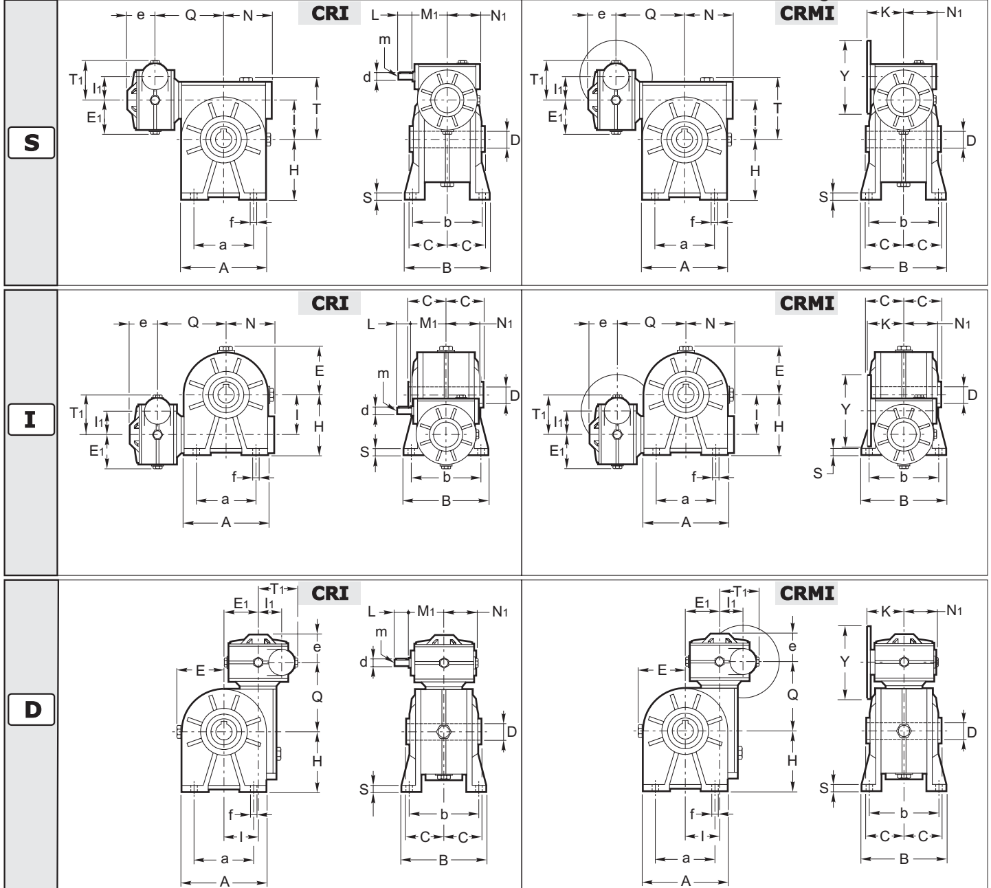
Dimensioni generali / Dimensions / Allgemeine Abmessungen
