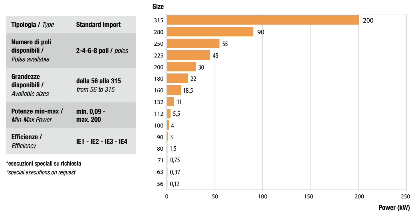
Grafico con taglie e valori di potenza massima in kW Chart with sizes and maximum power values in kW
